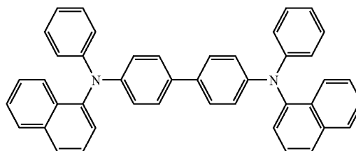
\alpha -NPD
